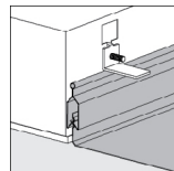
Versión de montaje por debajo con niveladores para techos SAS 150 154.
