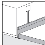
Versión de montaje por debajo con niveladores para techo de perfilera vista "T" 15/24mm.
