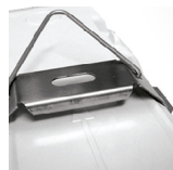
Pince de fixation avec triangle pour version suspendue
