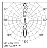
ELI 50 /W D/I 4000K 20° HO
