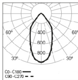
ELI /E 2 PB 4000K 60°
