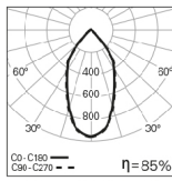
ELI Sq /W PB 4000K 60°
