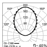
OREO Linea Up 1514mm bLINE 4000K
