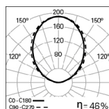
OREO Linea Up 1014mm bLINE 4000K
