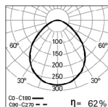
SPA/E LED gCONTROL+ 39W (590x590mm) 4000K
