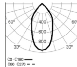
WEBB Spot /E 2 PB 4000K 60° LO
